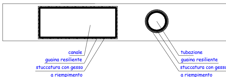
Figura 6-6: Passaggio dei canali e delle tubazioni attraverso elementi in cartongesso
